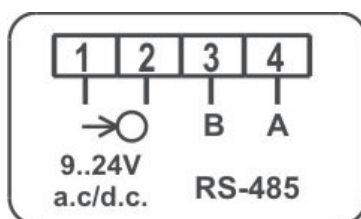
Sl. 2. Priključne sponke P19.
