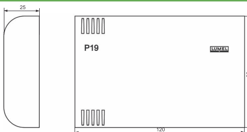
Sl.1. Obratovalni položaj in zunanje dimenzije
